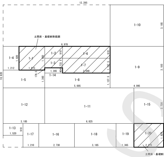
1階床 外皮面積等求積図
