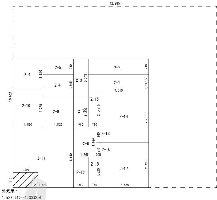
2階床 外皮面積等求積図
